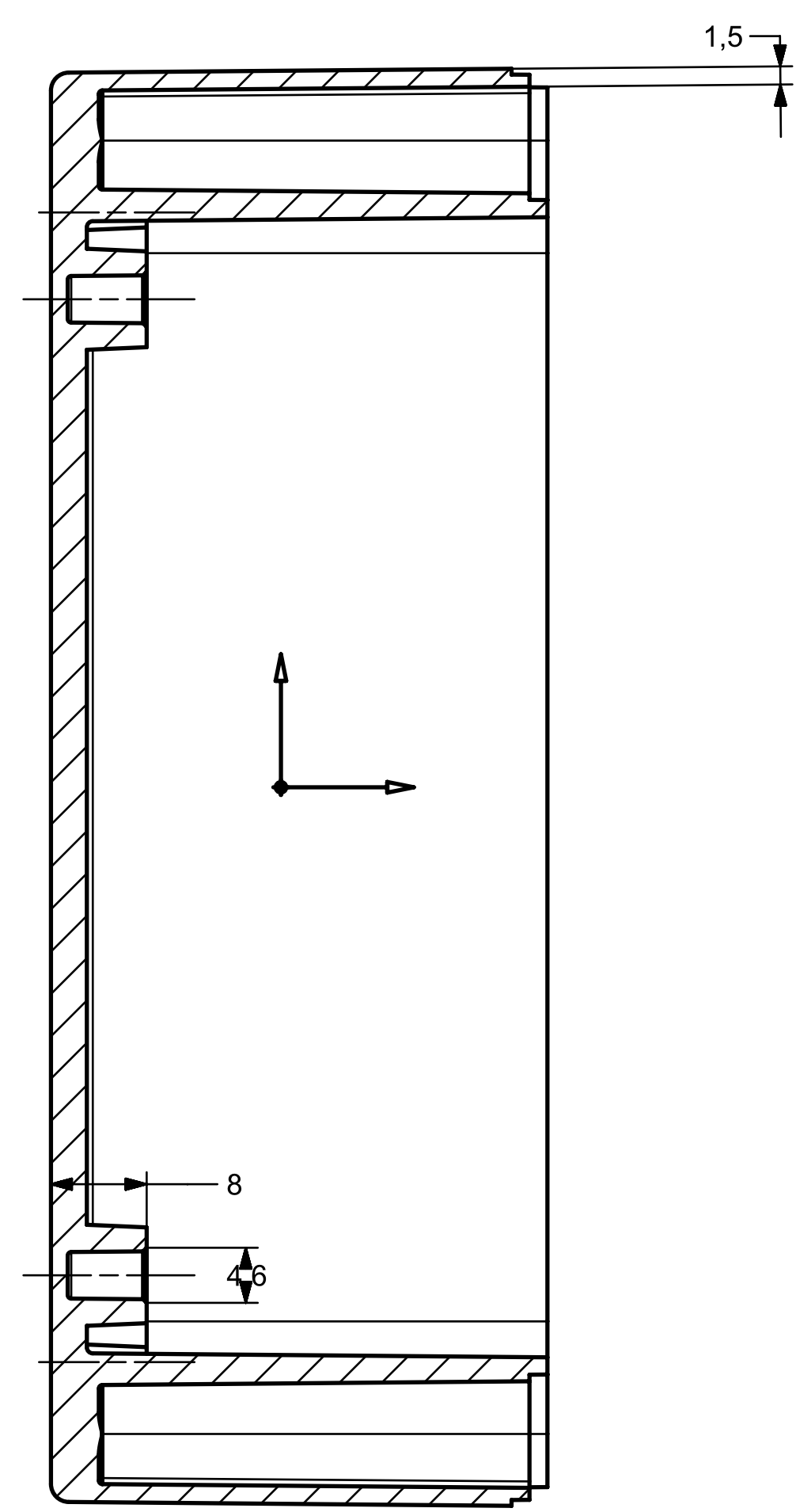
SECTION A-A
